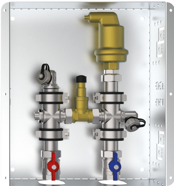
Strangentlüftung mit Warmhaltung
